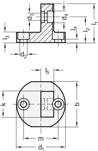
Kit de sujeción GN 511.1, Tipo K
